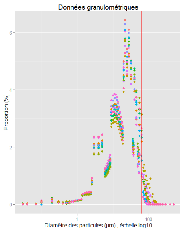
Figure 4 : Distribution granulométrique des échantillons de sédiment de l'étude préliminaire (n=12) (une couleur de point par échantillon, trait vertical rouge = 63 μm)
