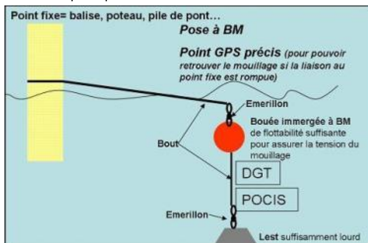
Figure 9. Exemple de mouillage "point-fixe"
