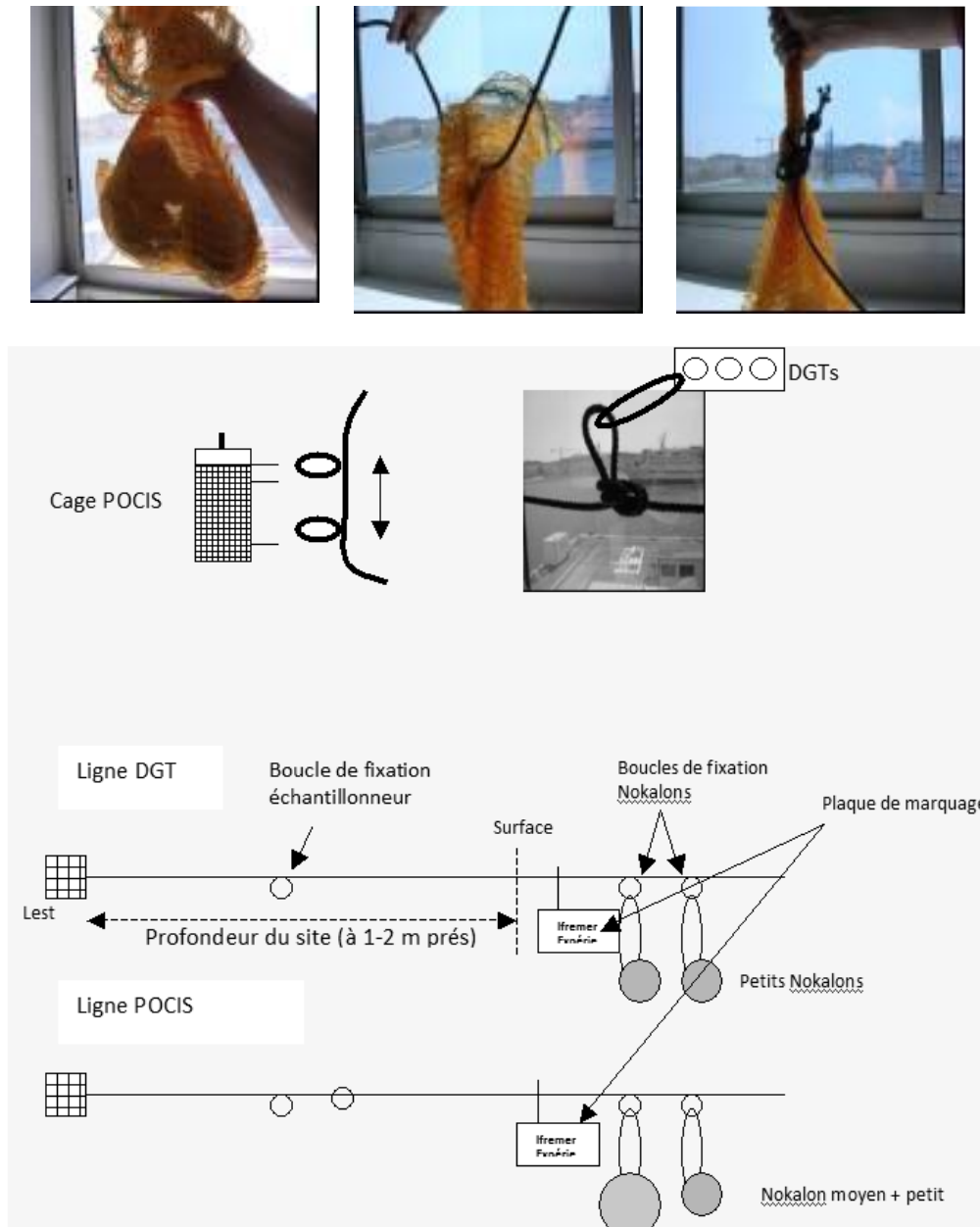
Figure 8. Exemple de lignes de mouillage pour POCIS et DGT
