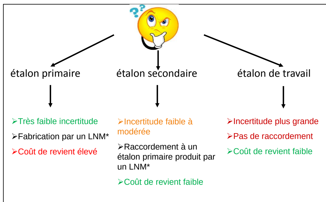
Figure 12 : Avantages et inconvénients des différents types d'étalons (LNM* : Laboratoire National de Métrologie)
